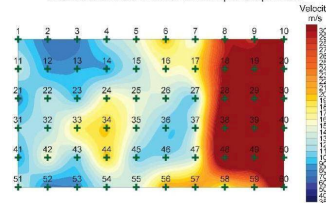
Distribuzione delle velocità soniche per trasparenza
